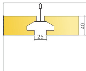
Løftplade kantdesign med svævende udseende.
