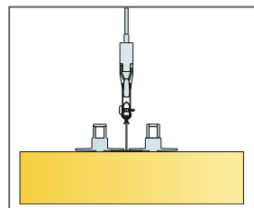
Montage mit T24 Hauptschiene
