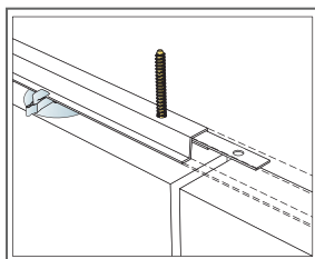
Connect profiiliin kiinnitys
