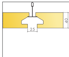
Plokštės įmontavimas plūduriuojančių lubų įvaizdžiui sudaryti
