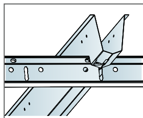
Profilijų sujungimas stabilizatoriaus kaiščiu
