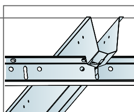
Profilų sujungimas stabilizatoriaus kaišiu
