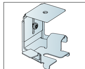
Detail Absorpční destičky. Minimální svěšeni systému 90-130mm.
