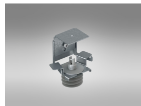
Függesztés Connect Absorber konzollal és Connect Absorber horgonnyal
