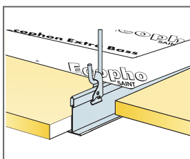
Suspensión con varilla y Clip de cuelgue
