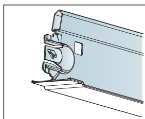
Dwarsprofiel PL
