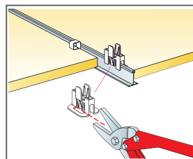
Stíhání Connect Hygiene klipu 20 pro inspekční panel
