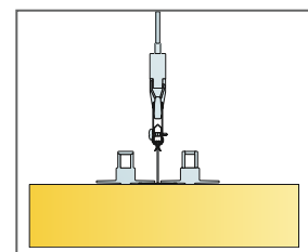
Montage med T24 Hovedprofil
