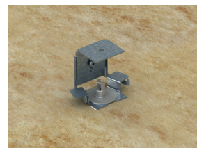
Nedhængning med Connect absorberent ophæng og Connect absorberent-anker
