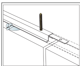
Infästning av Connect Skarvbleck för Baffleprofil
