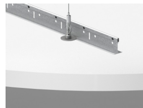
Solo Circle XL montage med Connect Absorbentankare
