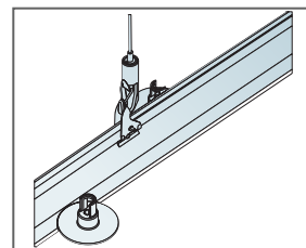
Installation med pendelfäste
