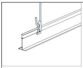
Kabinimas naudojant reguliuojamą kabinimo kablį ir fiksuatorių
