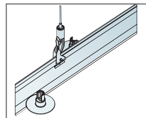
Kablio fikskatorių (hanger clips) montavimas
