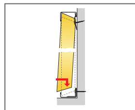
Asennusdetalji
