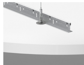
Solo Circle XL installatie met Connect Absorber anker
