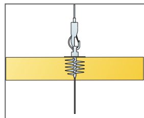
Panelen kunnen onder elkaar worden afgehangen
